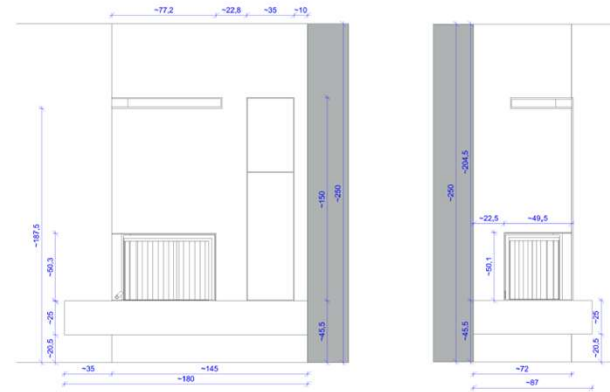
FUEGO alfarero Proyecto © Copyright: Carmina Borrera Nombre: P1 - ejemplo proyecto 3D Proyecto no: P1 - 2024 scale: 1:20 Date: 07.08.2024 El dibujo 3D se ha creado sobre la base de la información facilitada. No se garantiza ni se asume responsabilidad alguna por posibles errores de interpretación.
