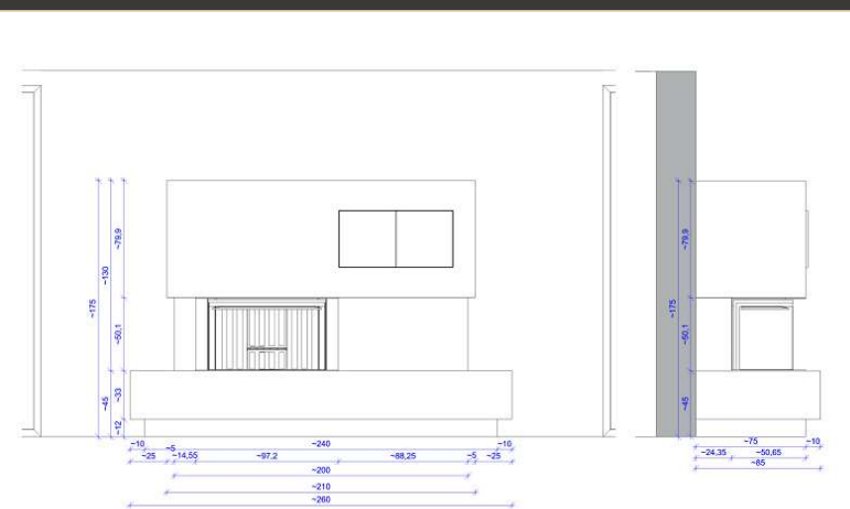
FUEGO el fuego Proyecto © Copyright Carmen Bañera Nombre: P2 EJEMPLO PROYECTO 3D Proyecto no.: P2 scale: 1:30 Date: 07.06.2024 Si desea 2D en su email o bien la copia de la información técnica, todos los derechos se reservan y quedan sujetos a modificaciones. No se permite su uso ni reproducción por medios electrónicos o impresos.
