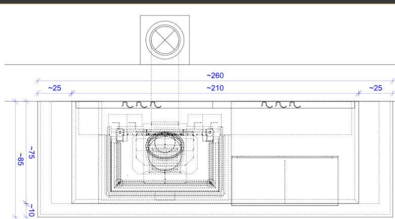
FUEGO el fuego Proyecto © Copyright Carmen Bañera Nombre: P2 EJEMPLO PROYECTO 3D Proyecto no.: P2 scale: 1:10 Date: 07.06.2024 Si desea 2D en su email o bien la copia de la información técnica, todos los derechos se reservan y quedan sujetos a modificaciones. No se permite su uso ni reproducción por medios electrónicos o impresos.
