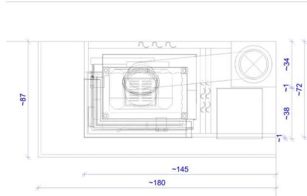
FUEGO alfarero Proyecto © Copyright: Carmina Borrera Nombre: P1 - ejemplo proyecto 3D Proyecto no: P1 - 2024 scale: 1:10 Date: 07.08.2024 El dibujo 3D se ha creado sobre la base de la información facilitada. No se garantiza ni se asume responsabilidad alguna por posibles errores de interpretación.
