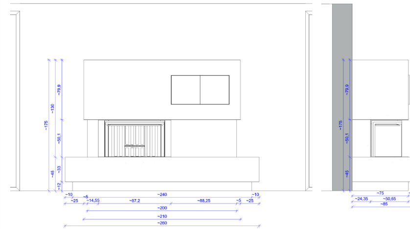
FUEGO elaboración Proyecto © Copyright: Carmen Bonora Nombre: P2 EJEMPLO PROYECTO 3D Proyecto no.: P2 scale: 1:20 Date: 07.06.2024 El dibujo 3D se ha creado sobre la base de la información facilitada, todos los dimensionados y detalles están contemplados detalladamente. No se aceptará ninguna responsabilidad por posibles errores y/o discrepancias.
