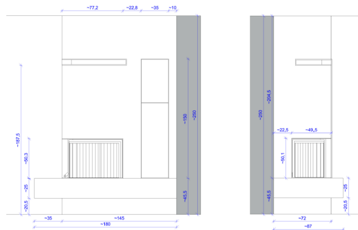
FUEGO difusión Proyecto 6 Copyright: Carmen Bonora Nombre: P1 - ejemplo proyecto 3D Proyecto no.: P1 - 2024 scale: 1:20 Date: 07.08.2024 El dibujo 2D se ha creado sobre la base de la información facilitada, sobre las dimensiones y detalles deben compararse cuidadosamente. No aceptamos ninguna responsabilidad por posibles errores u/o discrepancias.
