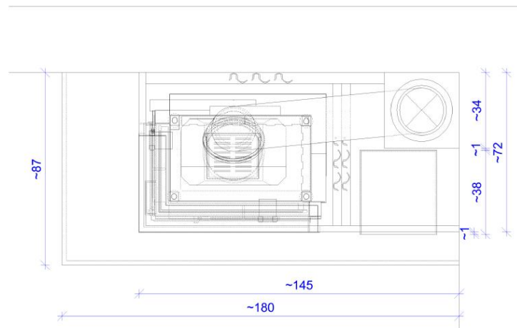
FUEGO difusión Proyecto 6 Copyright: Carmen Bonora Nombre: P1 - ejemplo proyecto 3D Proyecto no.: P1 - 2024 scale: 1:10 Date: 07.08.2024 El dibujo 2D se ha creado sobre la base de la información facilitada, sobre las dimensiones y detalles deben compararse cuidadosamente. No aceptamos ninguna responsabilidad por posibles errores u/o discrepancias.
